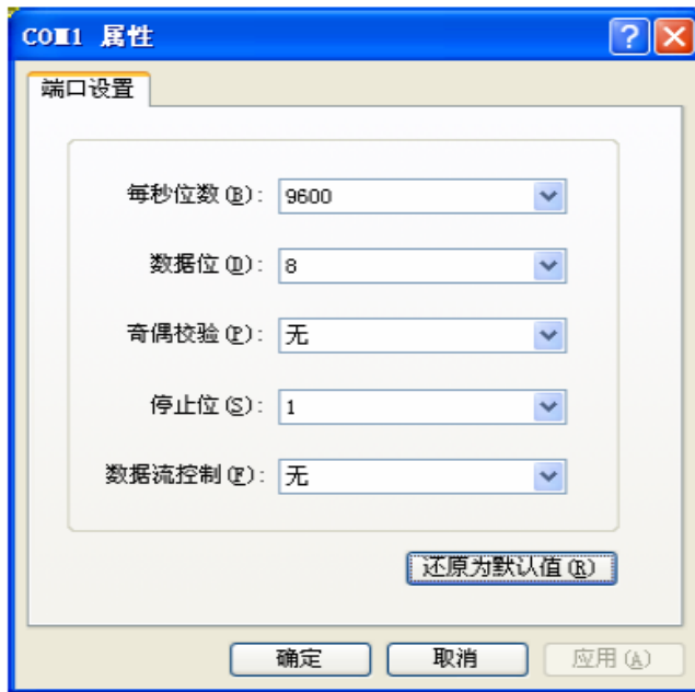
图 4 串口参数设置
