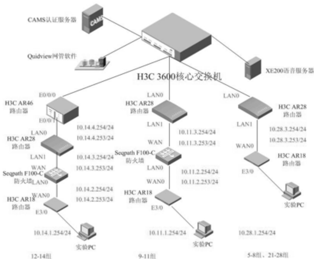
广东工业大学网络实验室拓扑示意图
